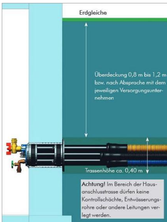
Bild 1: Maße Hauseinführung Keller
